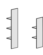
280x380xh1370 C 912 280x380xh1695 C 911
