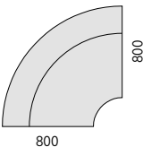
External high corner unit | Module d'angle externe haut
